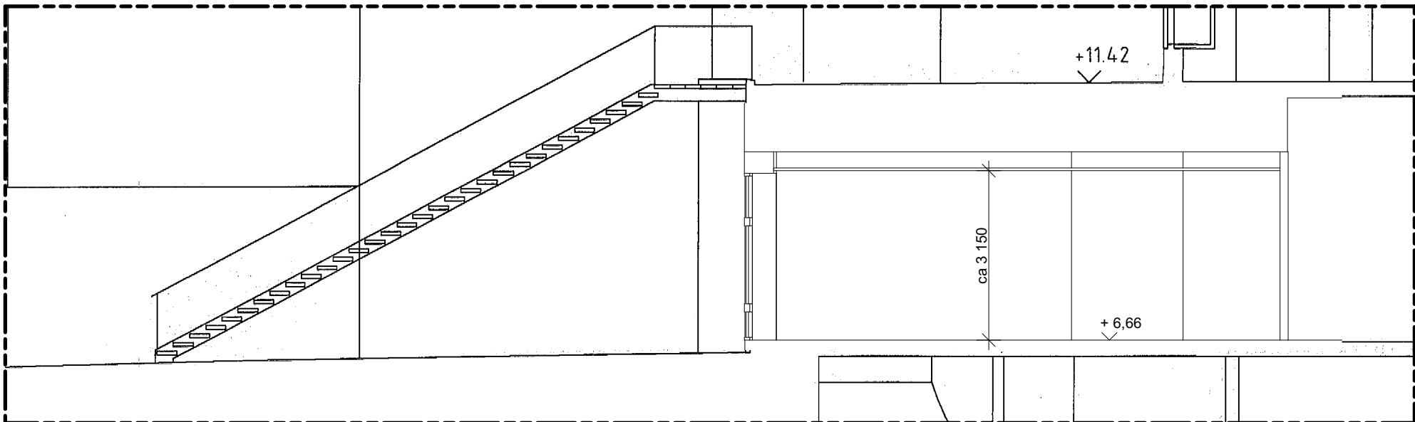
Sektion A skala: 1:100
